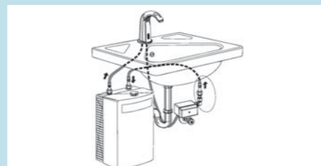
Dezentrale Warmwasserversorgung mit offenem Speicher
